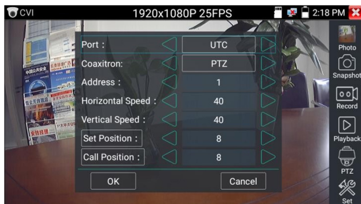
Рис.9 Настройки PTZ для видеокамер с UTC
